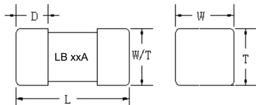
6-1 工程图（单位：mm） / Outline Drawing and Dimensions (Unit: mm)
