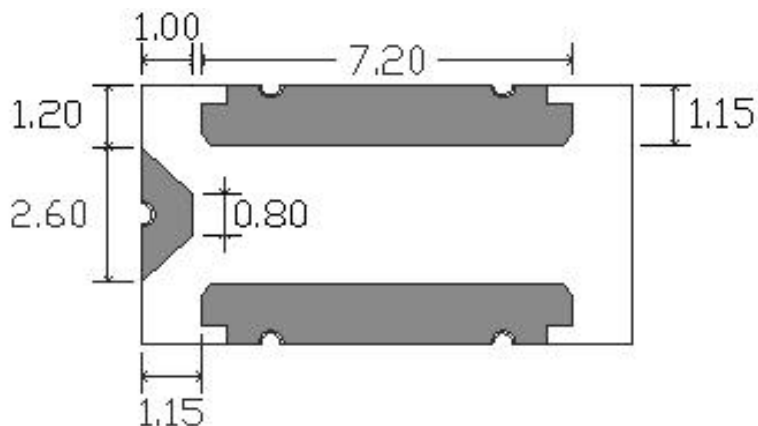
底视图 Bottom view
